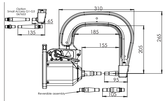
G3 - 022782 8 bar / 550 daN
