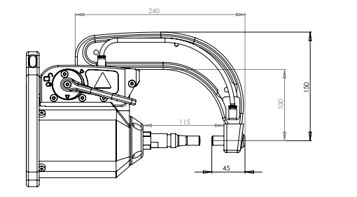
G6 - 022812 8 bar / 550 daN
