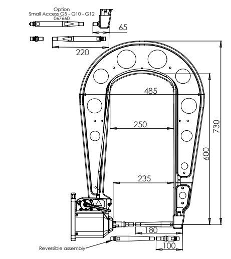
G5 - 022805 8 bar / 550 daN
