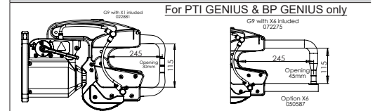
G9_X1 - 022881 8 bar / 550 daN G9_X6 - 072275 8 bar / 300 daN
