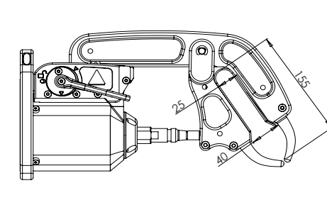
G7 - 022829 4 bar / 150 daN
