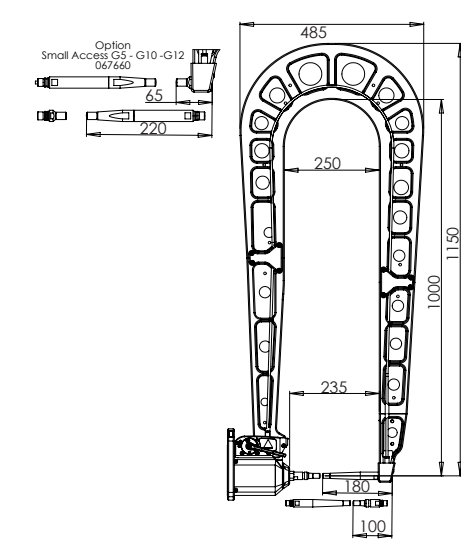
G12 - 075238 8 bar / 300 daN
