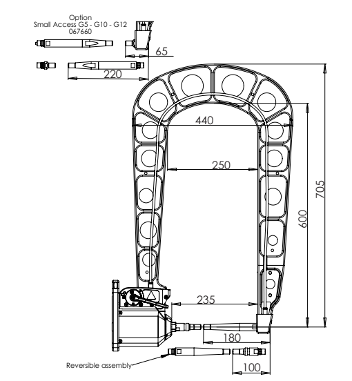
G10 - 067165 8 bar / 400 daN
