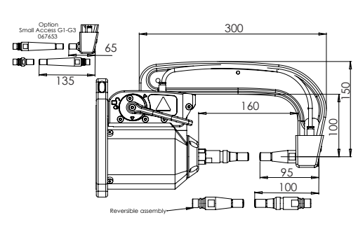
G1 - 022768 8 bar / 550 daN
