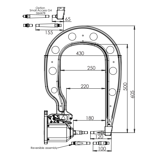
G4 - 022799 8 bar / 550 daN
