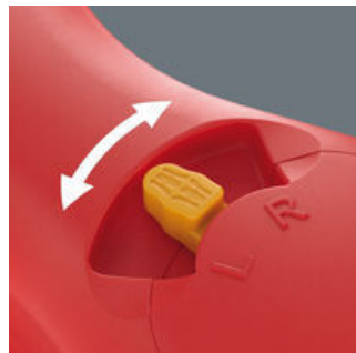
Die feinverzahnte Ratschenmechanik kann über einen Hebel leichtgängig in beide Richtungen umgeschaltet werden.
